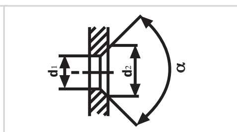
Bolt huls udførelse – konisk
