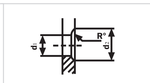
Bolt huls udførelse – sfærisk
