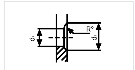
Bolt huls udførelse - sfærisk
